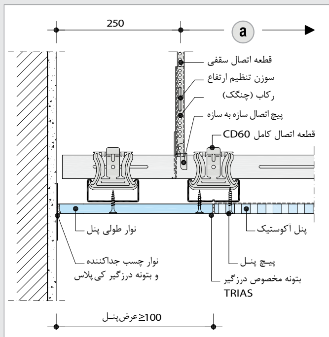
اتصال به دیوار بنایی با حاشیه ساده هم‌راستا با پنل آکوستیک
