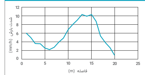
نمودار شدت پاشش آبپاش آلومینیومی تمام دور نازل ۱۰ و ۷ در فشار ۲ بار
