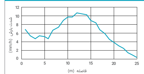
نمودار شدت پاشش آبپاش آلومینیومی تمام دور نازل ۱۰ و ۷ در فشار ۴ بار
