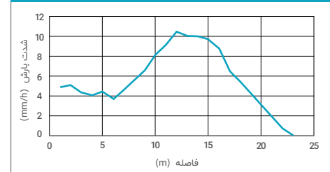
نمودار شدت پاشش آبپاش آلومینیومی تمام دور نازل ۱۰ و ۷ در فشار ۳ بار
